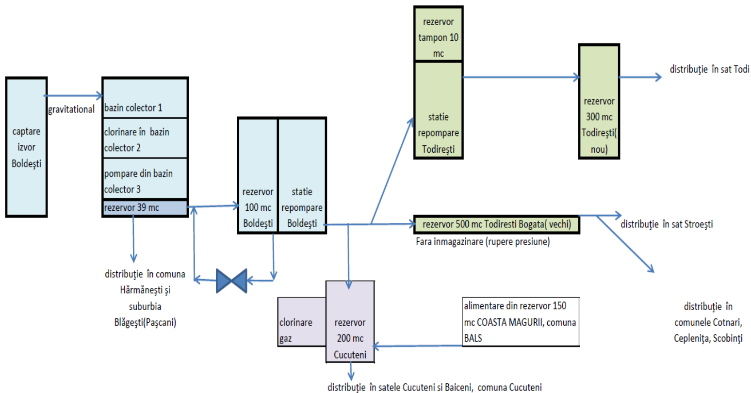
DIAGRAMA FLUX SISTEM APROVIZIONARE CU APA BOLDESTI
